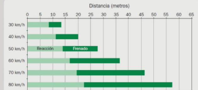
Figura 1.2 Ilustración de la distancia de detención en un frenado de emergencia
